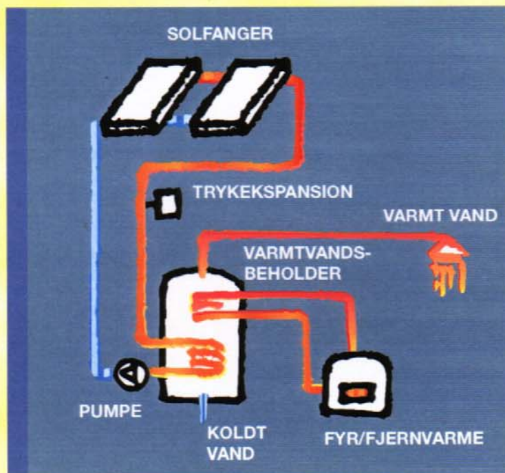
Principskitse af solvarmeanlæg
